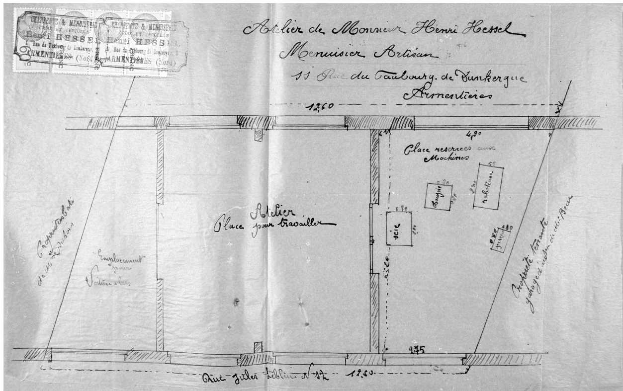
Scierie Henri Hessel, plan masse, 1922.
