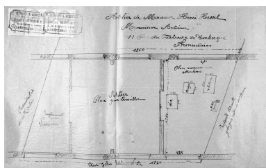
Scierie Henri Hessel, plan masse, 1922. Phot. Philippe Dapvril IVR31_19875902157X
