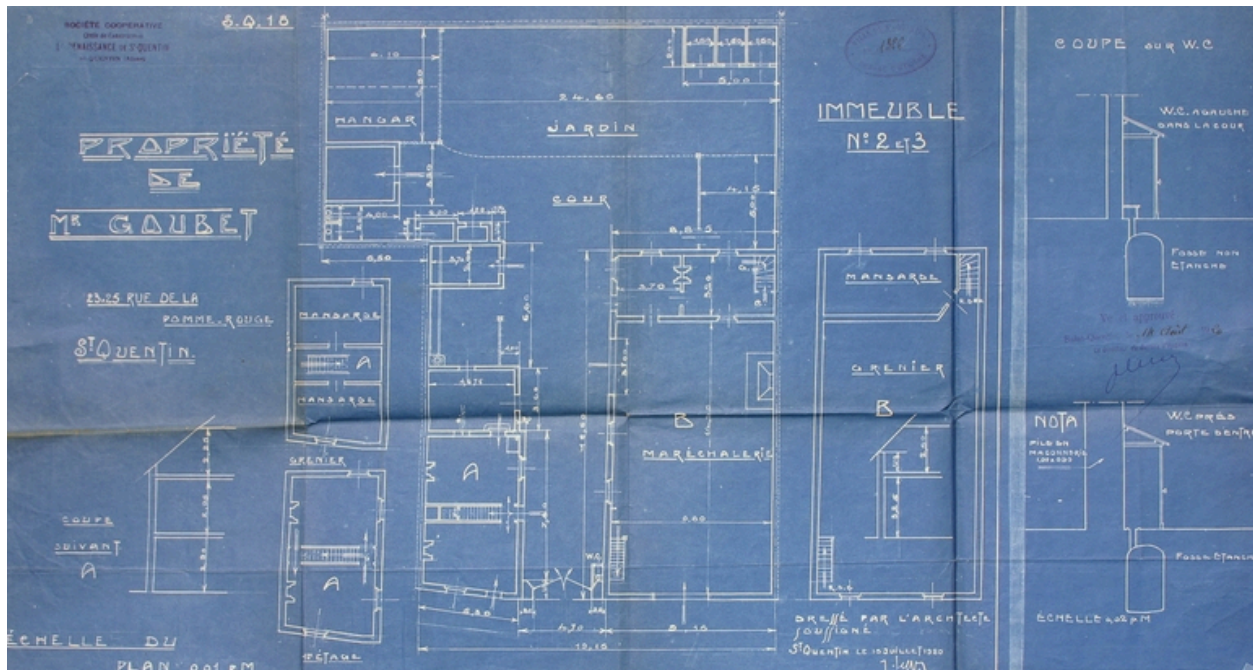
Plan de reconstruction des ateliers et logement de M. Goubet, 1920 (AC Saint-Quentin).
