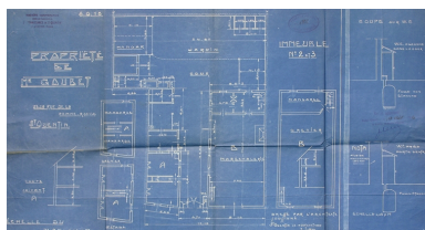
Plan de reconstruction des ateliers et logement de M. Goubet, 1920 (AC Saint-Quentin). Phot. Pillet Frédéric IVR22_20060205571NUCAB
