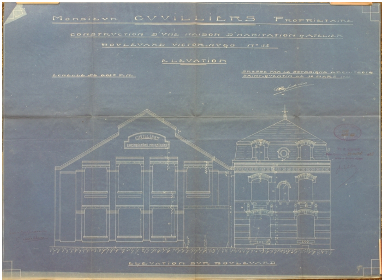
Façade sur boulevard, 1923, par Carpentier (AC Saint-Quentin).
