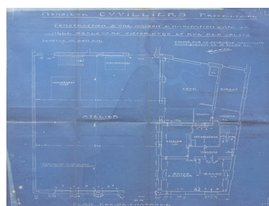
Plan du rez-de-chaussée, 1923, par Carpentier (AC Saint-Quentin).
