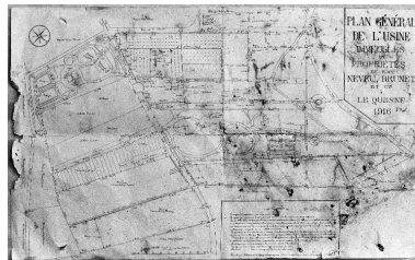
Plan générale de l'usine, 1916 (AP). Phot. Benoît Dufournier (reproduction) IVR22_19878000410ZB
