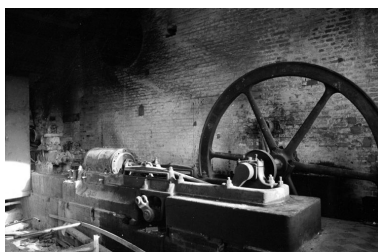
Salle des machines, élévation antérieure, machine à vapeur. Phot. Benoît Dufournier IVR22_19878000418Z
