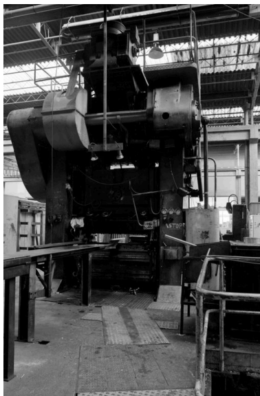
CLAIROIX. Usine d'emboutissage Gantois. Machine de production. Phot. Benoît Dufournier IVR22_19936002404Z
