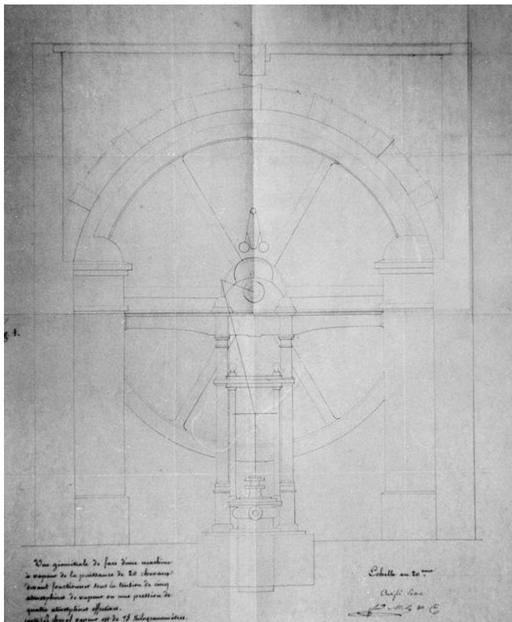
BERNEUIL. Vue générale de face d'une machine à vapeur de la puissance de 20 chevaux, 1852 (AD Oise ; série 5M).
