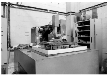
CLAIROIX. Usine d'emboutissage Gantois. Machine de production. Phot. Benoît Dufournier IVR22_19936002410Z
