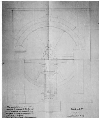
BERNEUIL. Vue générale de face d'une machine à vapeur de la puissance de 20 chevaux, 1852 (AD Oise ; série 5M). Phot. Benoît Dufournier IVR22_19936001602ZB
