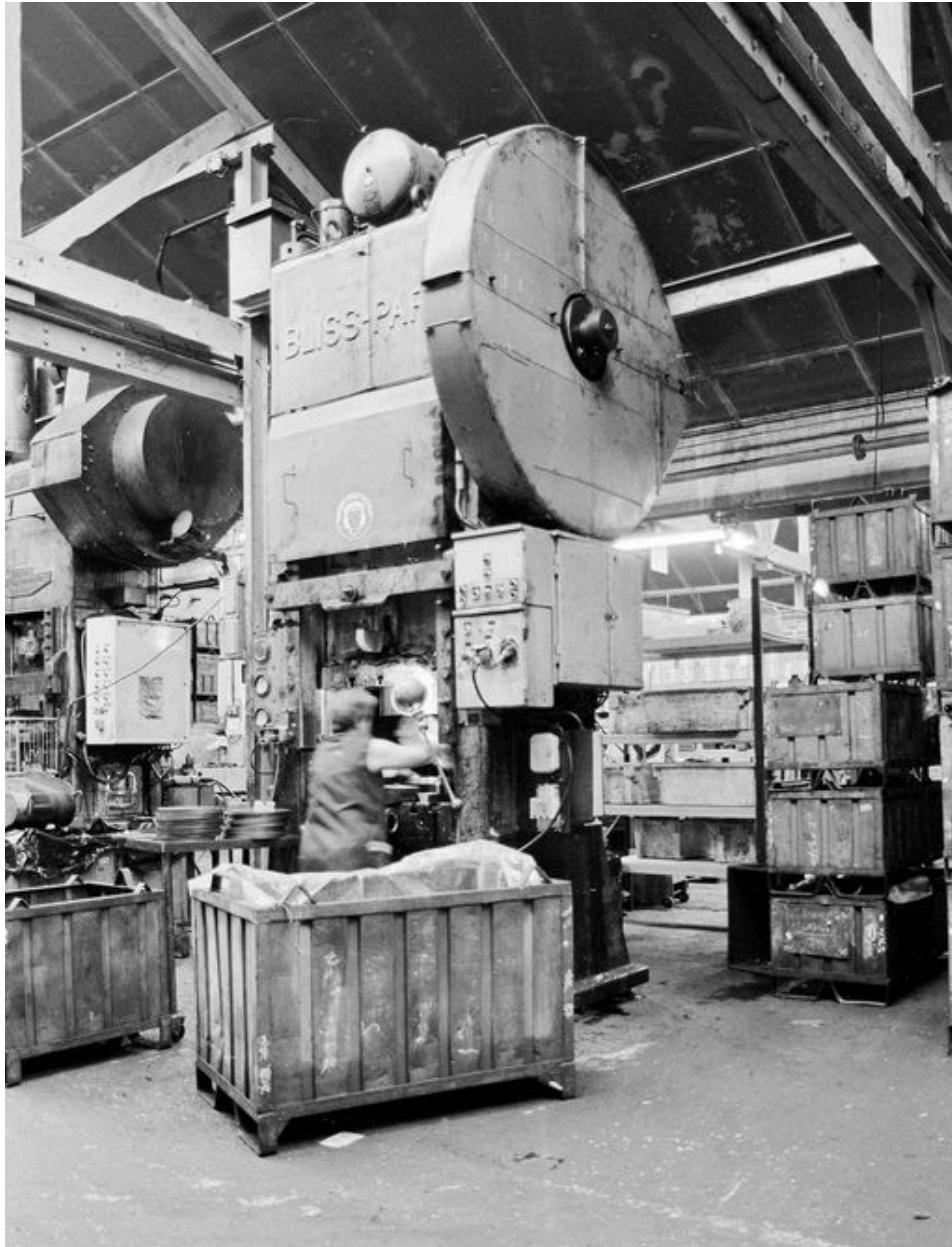
CRISOLLES. Usine de construction mécanique Lelong puis usine de roulements M.P.R. : presse d'emboutissage.
