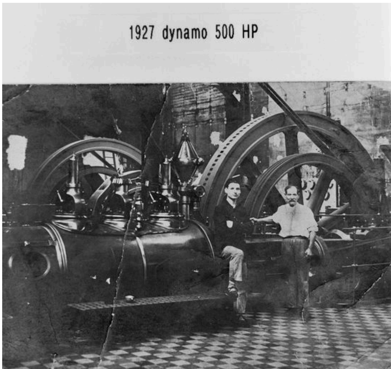
TROSLY-BREUIL. Usine de produits chimiques dite de Cuise-Lamotte ou de Lamotte-Breuil, puis Socindus. Machine à vapeur, en 1927 (AP).
