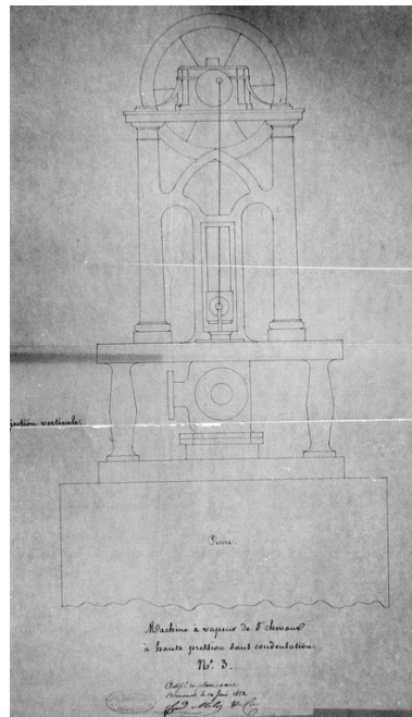
BERNEUIL. Vue en coupe d'une machine à vapeur à haute pression de 5 chevaux sans condensation, 1852 (AD Oise ; série 5M). Phot. Benoît Dufournier IVR22_19936001604ZB
