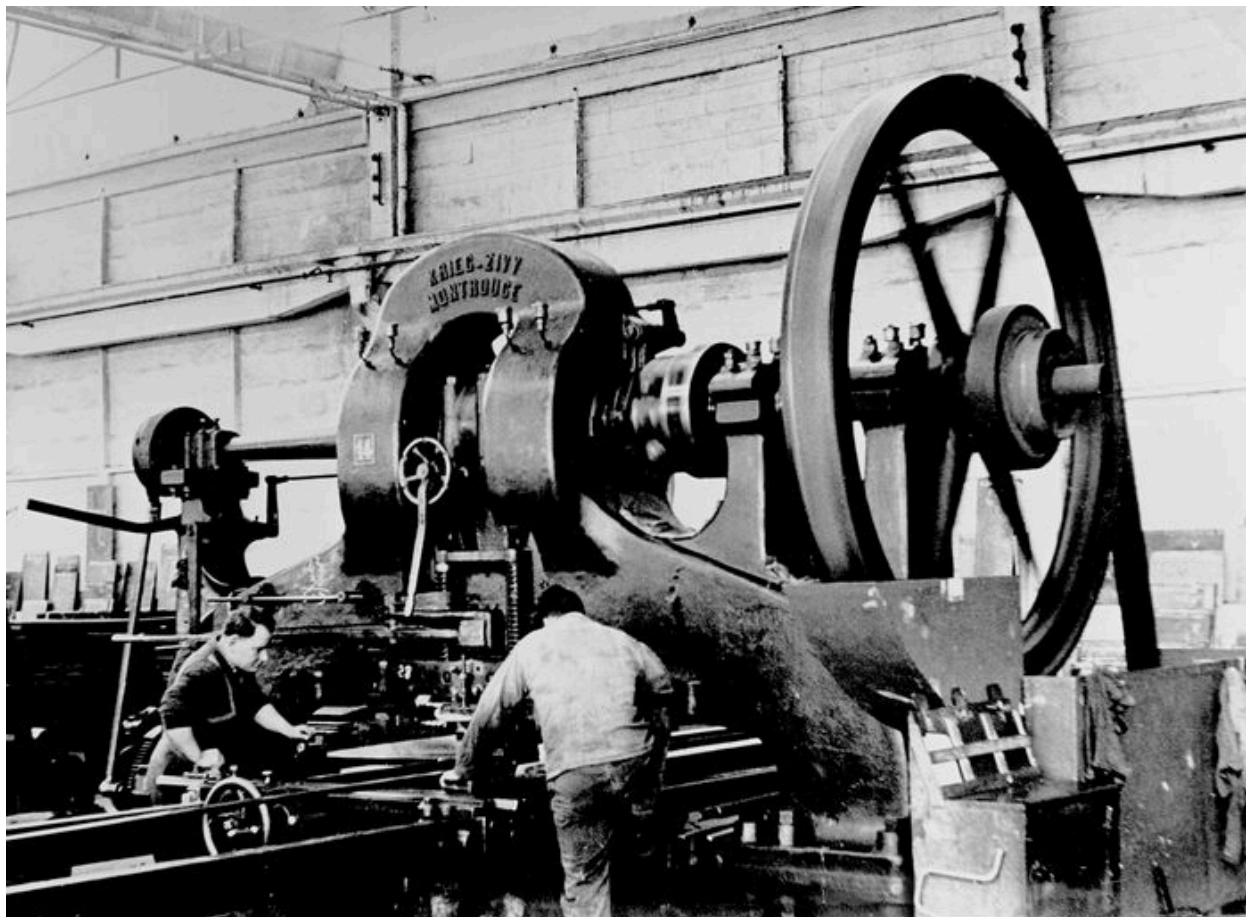
CHEVRIERES. Usine de chaudronnerie Krieg et Zivy. Ouvriers au travail sur une machine Krieg et Zivy de Montrouge (AP).
