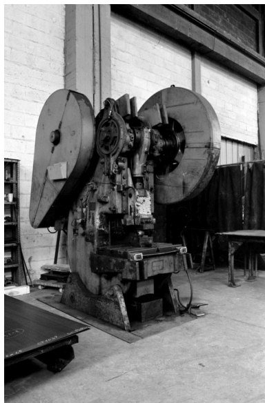
CLAIROIX. Usine d'emboutissage Gantois. Machine de production. Phot. Benoît Dufournier IVR22_19936002406Z
