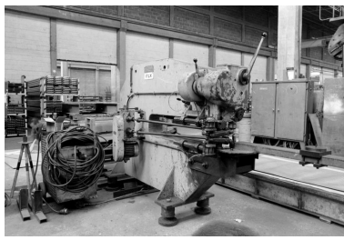
CLAIROIX. Usine d'emboutissage Gantois. Machine de production. Phot. Benoît Dufournier IVR22_19936002401Z
