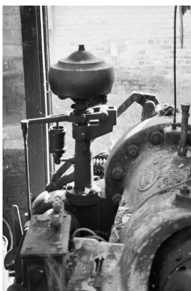
LA CROIX-SAINT-OUEN, Moteur à pistons à combustion (machine à pression d'huile) du constructeur Duvant, installé dans l'ancienne usine de jouets en bois. Monart Phot. Bertrand Fournier IVR22_20006000695Z
