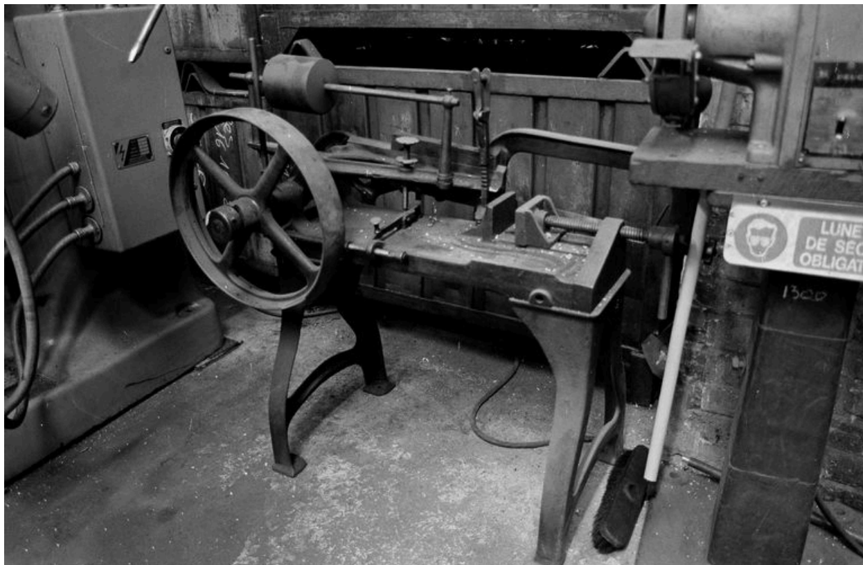
CRISOLLES. Usine de construction mécanique Lelong puis usine de roulements M.P.R. : machine destinée à scier les rondins de fer (?)
