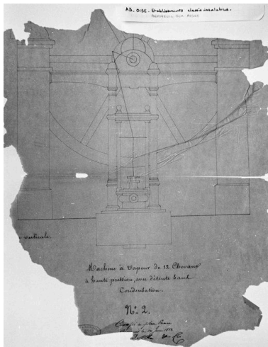
BERNEUIL. Machine à vapeur de 12 chevaux à haute pression avec détente sans condensation, 1852 (AD Oise ; série 5M). Phot. Benoît Dufournier IVR22_19936001603ZB
