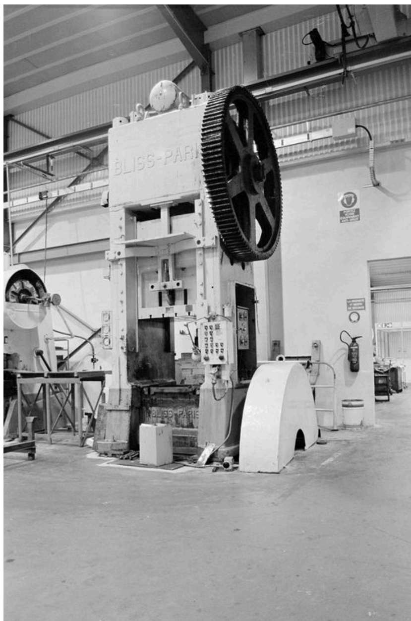
CRISOLLES. Usine de construction mécanique Lelong puis usine de roulements M.P.R. : presse mécanique du constructeur Bliss.
