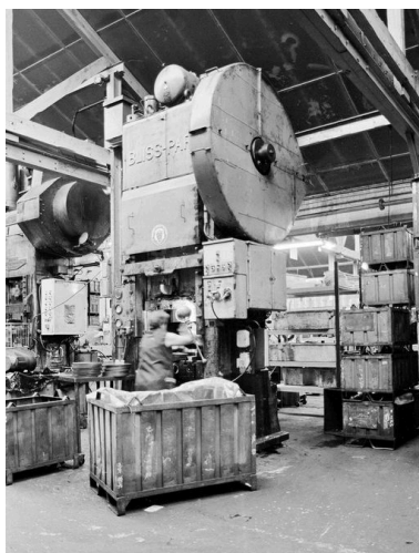
CRISOLLES. Usine de construction mécanique Lelong puis usine de roulements M.P.R. : presse d'emboutissage. Phot. Benoît Dufournier IVR22_19936001645Z
