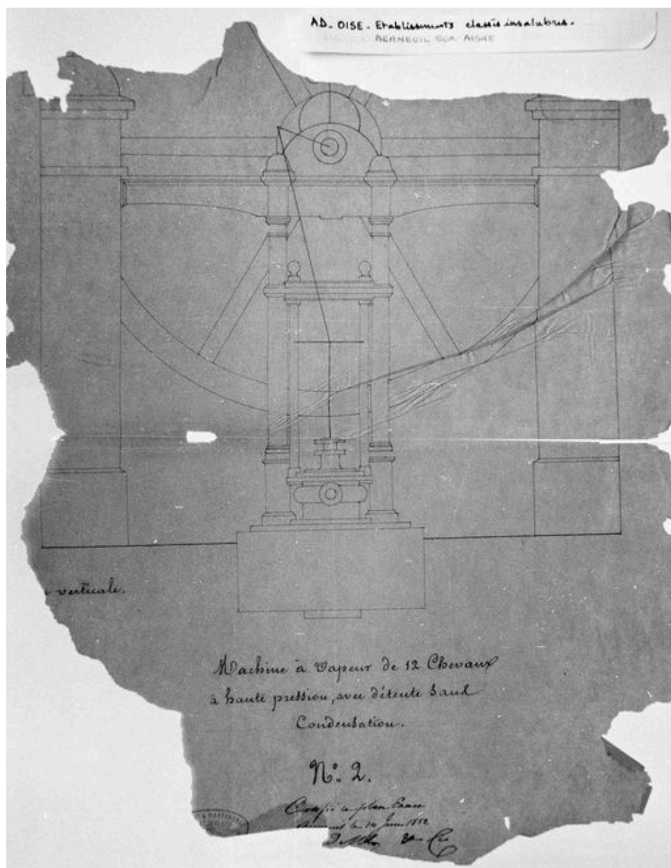
BERNEUIL. Machine à vapeur de 12 chevaux à haute pression avec détente sans condensation, 1852 (AD Oise ; série 5M).
