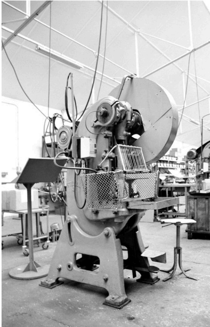
CRISOLLES. Usine de construction mécanique Lelong puis usine de roulements M.P.R. : presse d'emboutissage et de rivetage.
