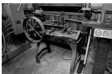
CRISOLLES. Usine de construction mécanique Lelong puis usine de roulements M.P.R. : machine destinée à scier les rondins de fer (?) Phot. Benoît Dufournier IVR22_19936001646Z
