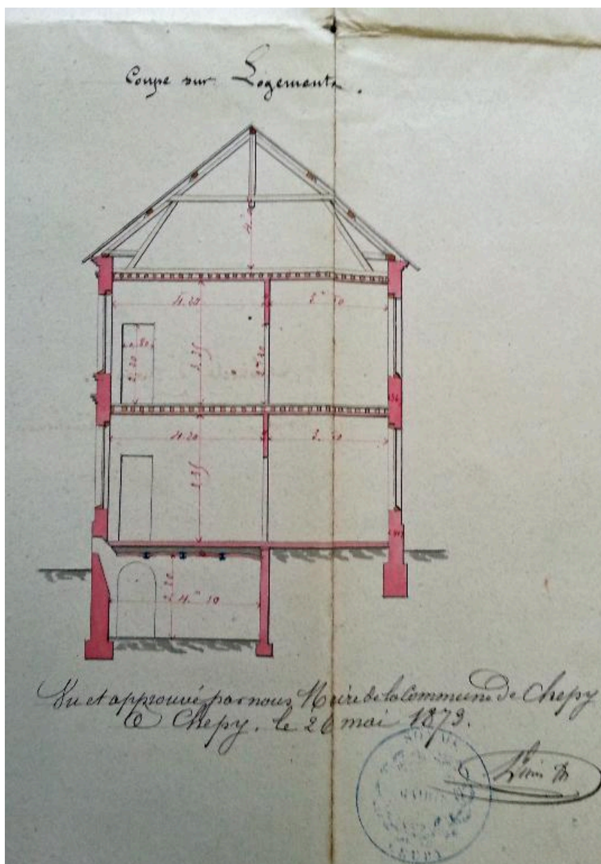
Plan de coupe des logements, dressé par l'architecte Delignères, en 1873 (AD Somme ; 99 O 1145).
