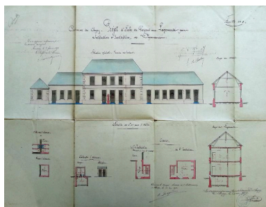
Plans dressés par l'architecte Delignères, 1873 (AD Somme ; 99 O 1145). Phot. Romain Grimaud (reproduction) IVR22_20138015842NUCA
