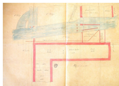
Plan détaillé des moulins de Beaupré, 1855 (AD Oise, 7 Sp 142). Phot. Fournier Bertrand (reproduction) IVR22_20036000007NUCAB
