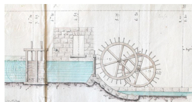
Profil du moulin de Beaupré annexé au rapport sur l'usine du sieur Philippe, 23 septembre 1836 (AD Oise ; 7 Sp 142). Phot. Fournier Bertrand (reproduction) IVR22_2003600003NUCAB
