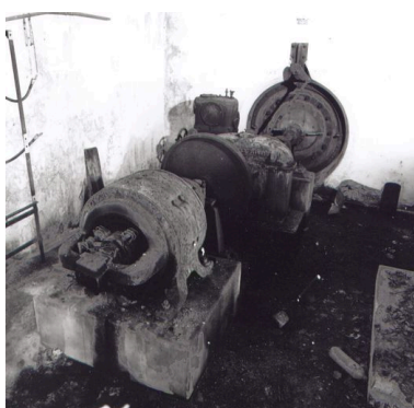
Intérieur de la salle des machines, détail de l'inscription de l'entrepreneur Alternateur Gramme, vue d'ensemble. Phot. Thierry Lefébure IVR22_20026000765X
