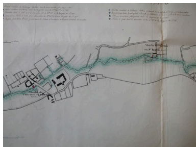
Plan d'ensemble des moulins de Thérines, annexe au projet de règlement des moulins, 24 novembre 1837.
