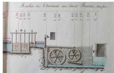
Profil du moulin de Thérines, au sieur Boniface Breton annexe au projet de règlement des moulins de Thérines, 24 novembre 1837.
