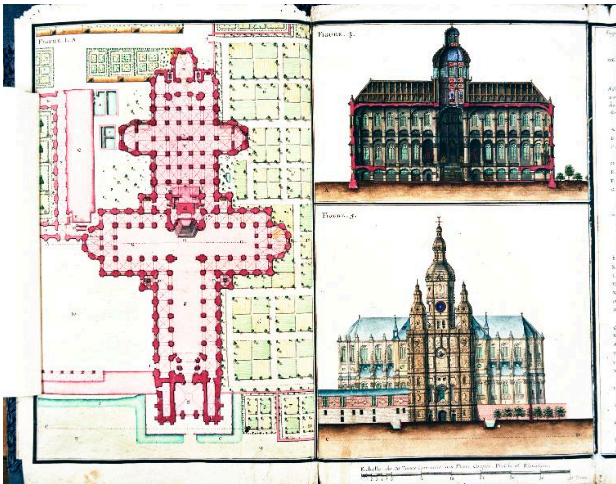
Plan, élévation et coupe de l'église abbatiale de Saint-Amand, Claude Masse, 1725 (Ministère de la Défense, SHD, Vincennes, Fonds du Génie, Atlas Ms 131k, f°84).
