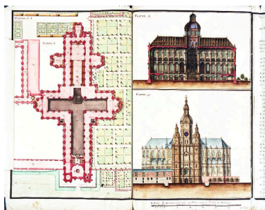
Plan du sous-sol (niveau de la crypte), élévation et coupe de l'église abbatiale de Saint-Amand, Claude Masse, 1725 (Ministère de la Défense, SHD, Vincennes, Fonds du Génie, Atlas Ms 131k, f°84). Phot. Dapvril Philippe IVR31_19935900389XE
