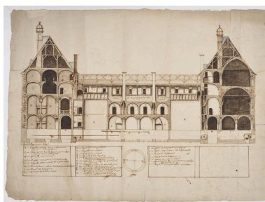
Coupe de l'aile est du cloître de l'abbaye, vers 1700 (Musée municipal Saint-Amand-les-Eaux). IVR31_20135908052NUCA
