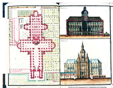
Plan, élévation et coupe de l'église abbatiale de Saint-Amand, Claude Masse, 1725 (Ministère de la Défense, SHD, Vincennes, Fonds du Génie, Atlas Ms 131k, f°84). Phot. Dapvril Philippe IVR31_19935900388XE
