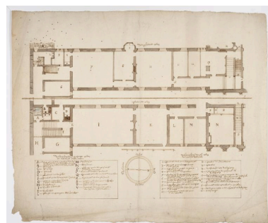
Plan du rez-de-chaussée et du premier étage du quartier abbatial, vers 1700 (Musée municipal Saint-Amand-les-Eaux). IVR31_20135908059NUCA
