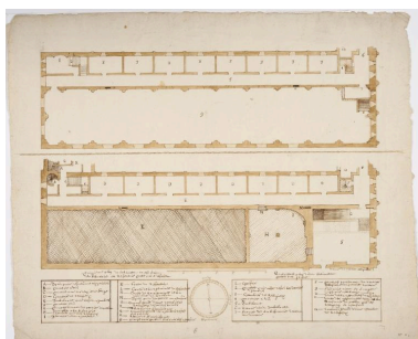
Plan du 3e et 4e étage du cloître, vers 1700 (Musée municipal Saint-Amand-les-Eaux). IVR31_20135908058NUCA
