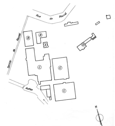
Schéma de situation : A. Bureau, B. Magasin industriel, C. Ateliers de fabrication, D. Logement patronal. Dess. Marie-Laure Monnehay-Vulliet, Autr. Stéphane Gonet IVR32_20168000762NUD
