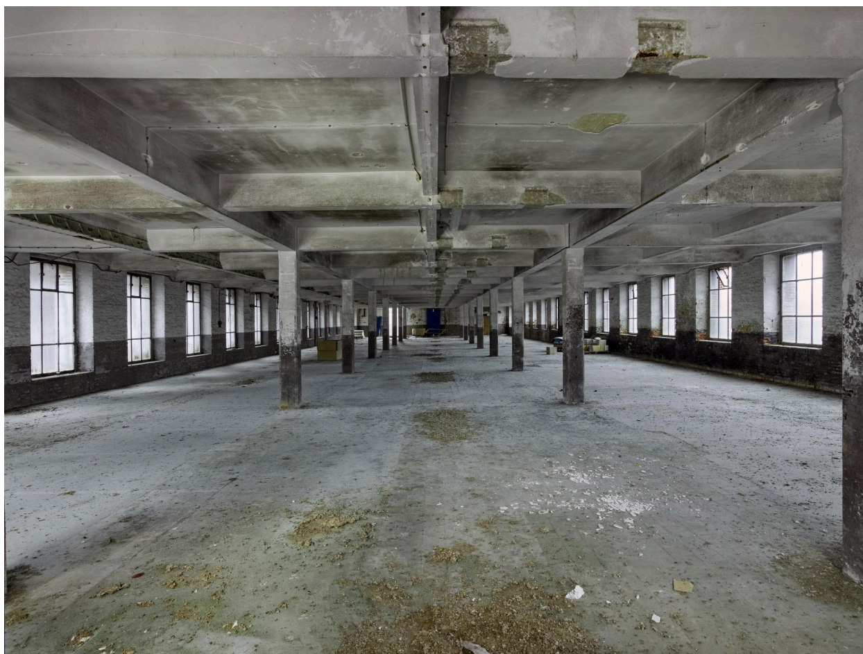
Vue intérieure longitudinale du premier étage en béton de l'atelier de fabrication (bâtiment A).
