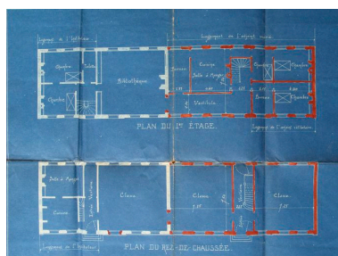
Plans du rez-de-chaussée et du premier étage par Anatole Bienaimé, 1903 (AD Somme ; 99 O 680). Phot. Fournier Bertrand (reproduction) IVR22_20088015019NUCA
