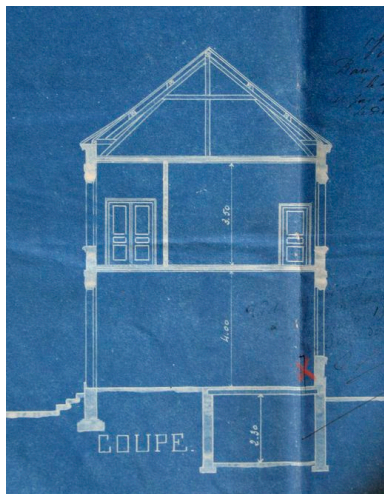
Coupe transversale par Anatole Bienaimé, 1903 (AD Somme ; 99 O 680). Phot. Fournier Bertrand (reproduction) IVR22_20088015020NUCA
