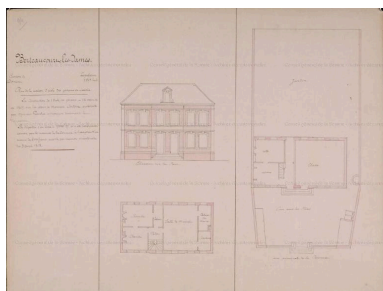
Berteaucourt-les-Dames. Plan de la nouvelle maison d'école de garçons et mairie, 1878 (AD Somme ; 99 T 3804 94/2). Phot. Archives départementales de la Somme (reproduction) IVR22_20138016162NUC2A
