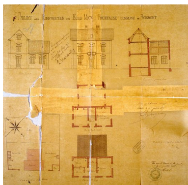
Plan, coupe et élévation du projet de l'école de Pinchefalise en 1877. Phot. Monnehay-Vulliet Marie-Laure IVR22_20068000078XAB
