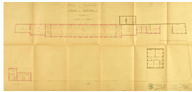
Ville de Bapaume, École de garçons - projet. Dessin aquarellé plan du premier étage. Signé et daté L. Roussel, 15 décembre 1908 et 8 mars 1909. (AD Pas-de-Calais, 20612/1). Phot. Pierre Thibaut IVR32_20216200300NUCA
