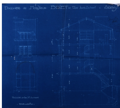
Arras. Propriété de M. Briet, 19 rue Saint-Aubert. Façade sur la rue Saint-Aubert, 1929 (AD Pas-de-Calais).
