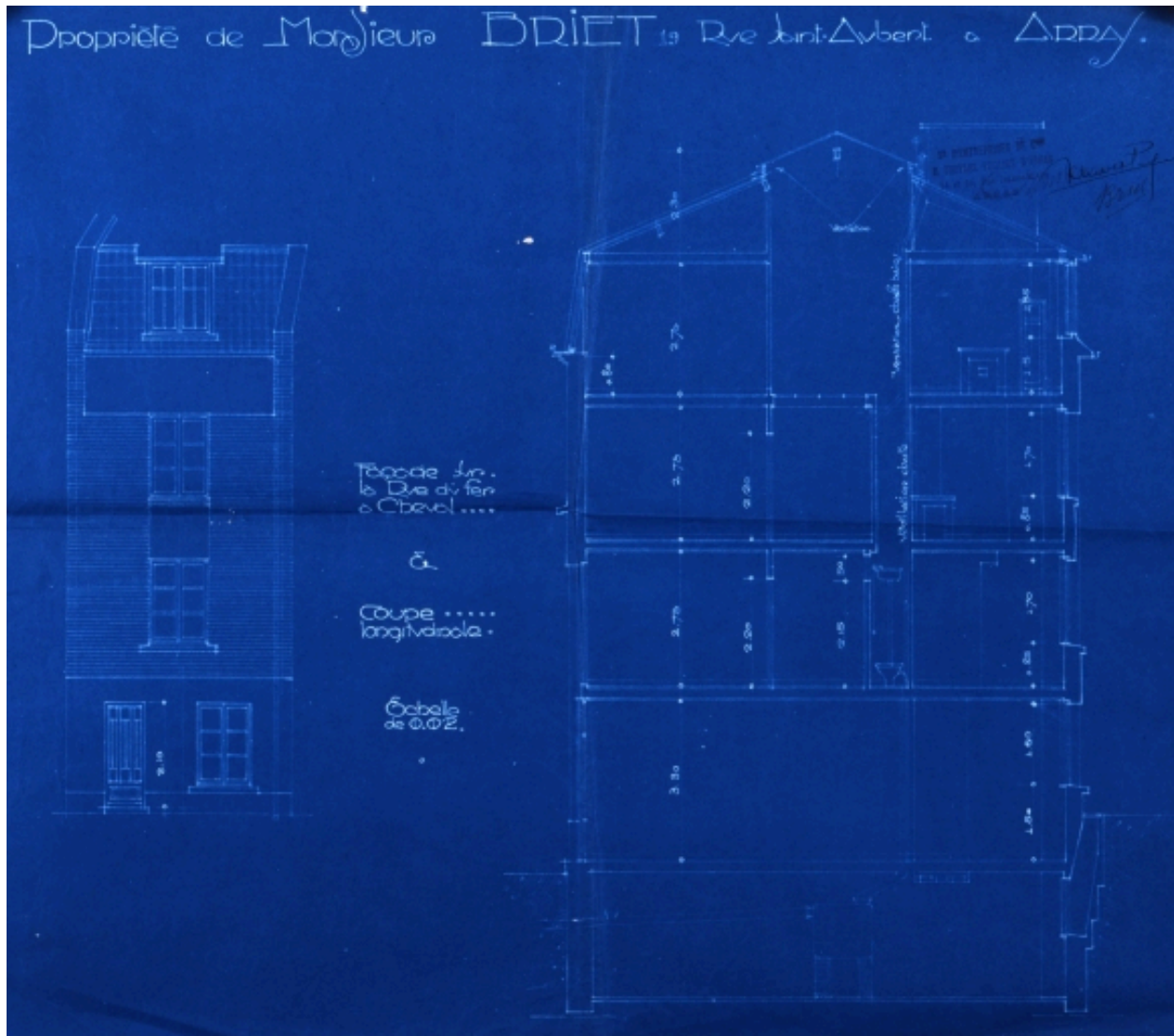
Arras. Propriété de M. Briet, 19 rue Saint-Aubert. Façade sur la rue du Fer-à-Cheval, 1929 (AD Pas-de-Calais).
