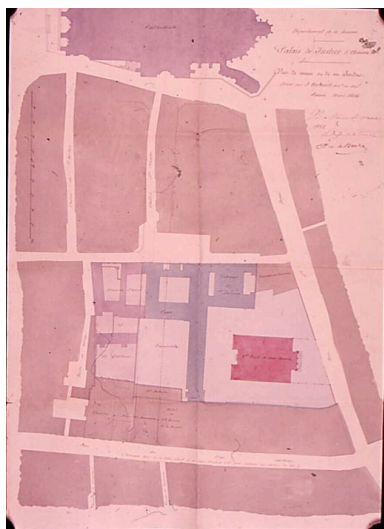
Plan de masse des abords du palais de justice (ancien couvent de célestins), 1856 (AD Somme ; 99 N 136928). Phot. Archives départementales de la Somme (reproduction) IVR22_20048010924NUCA
