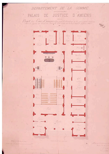
Palais de justice d'Amiens. Projet (non réalisé) de cour d'assises, 1860 (AD Somme ; 99 N 136928). Phot. Archives départementales de la Somme (reproduction) IVR22_20048010925NUCA
