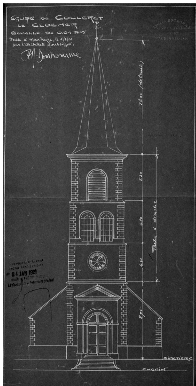
Projet non réalisé de restauration de l'église de Colleret par l'architecte Armand Bonhomme. Plan, 1920 (AD Nord ; 149 O 144).
