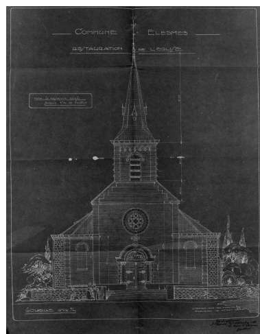
Projet non réalisé de restauration de l'église d'Élesmes par les architectes Afchain et Mereau, 1923 (AD Nord ; 188 O 70). Phot. Thierry Petitberghien IVR31_20015902495X
