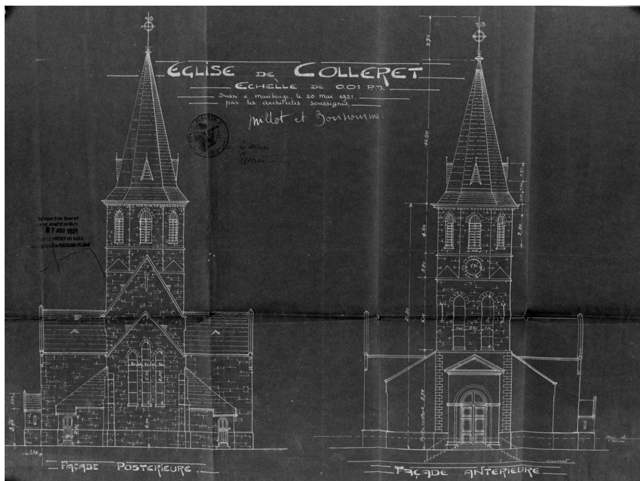
Projet de restauration de l'église de Colleret par les architecte Milot et Bonhomme. Plan, 1921 (AD Nord ; 149 O 144).
