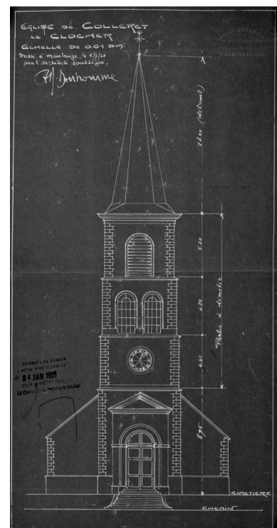
Projet non réalisé de restauration de l'église de Colleret par l'architecte Armand Bonhomme. Plan, 1920 (AD Nord ; 149 O 144). Phot. Thierry Petitberghien IVR31_20015901955X
