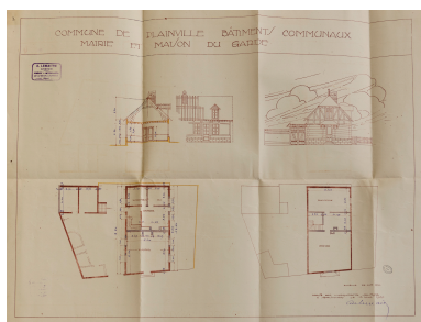
Plan de la mairie à reconstruire avec maison du garde, A. Lemaître, 1920 (AD Oise ; 2 O 11596). Repro. Marc Kérignard IVR32_20246000058NUCA
