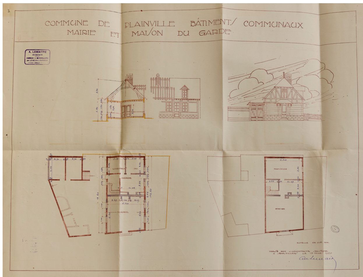
Plan de la mairie à reconstruire avec maison du garde, A. Lemaître, 1920 (AD Oise ; 2 O 11596).
