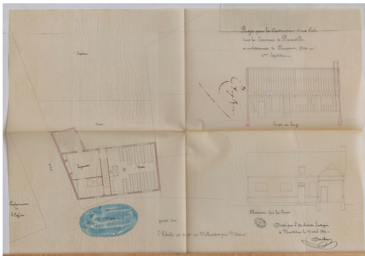
Plan pour le projet de construction d'une école, D. Dercheu, 1839, (AD Oise ; 2 O 11585).
