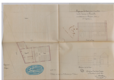
Plan pour le projet de construction d'une école, D. Dercheu, 1839, (AD Oise ; 2 O 11585). Repro. Marc Kérignard IVR32_20246000062NUCA
