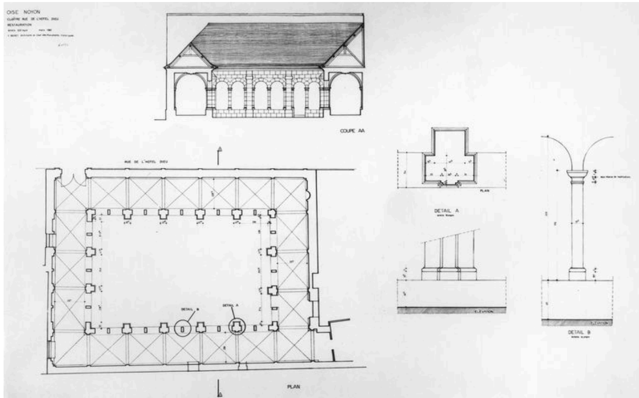
Relevé du cloître par Boiret, 1982 (Médiathèque du Patrimoine ; carte à fenêtre 60152).
