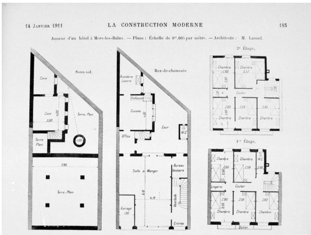
Annexe d'un hôtel à Mers-les-Bains. Plans. Architecte M. A Lasnel. La Construction moderne, 1911 (AD Somme ; 1 J 3584/10).
