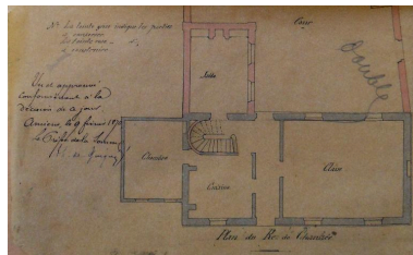
Saint-Ouen. Projet d'agrandissement du logement de l'instituteur et construction d'une salle de mairie. Plan, Antoine architecte, 1869 (AD Somme ; 99 O 3405). Phot. Isabelle Barbedor IVR22_20108010149NUCA
