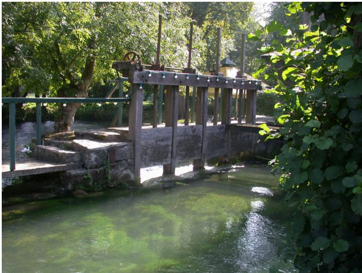
Les vannes de décharge et le repère de niveau des eaux.
