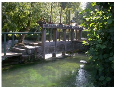
Les vannes de décharge et le repère de niveau des eaux. Phot. Bertrand Fournier IVR22_20026000870NUCA
