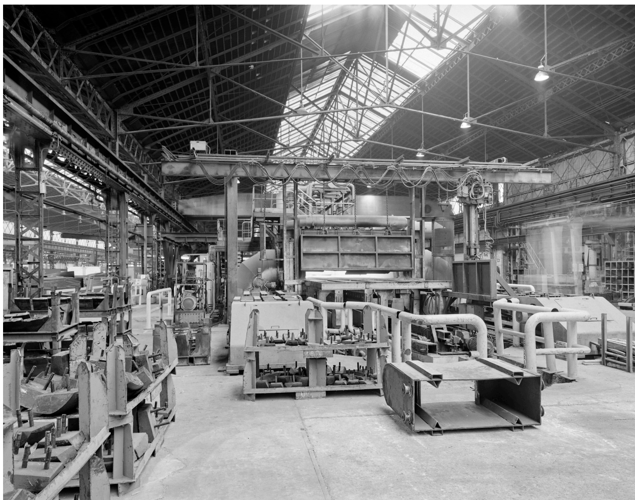
Hall 7 : le four de la presse de 1 500 tonnes. Vue de face.
