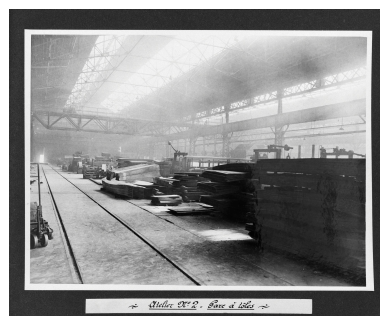
Atelier n° 2 : parc à tôles, 16 février 1940. Photographe inconnu (coll. part., archives Cerec). Repro. Thierry Petitberghien IVR31_20025900604XB
