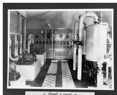
Centrale à mazout, 16 février 1940. Photographe inconnu (coll. part., archives Cerec).
