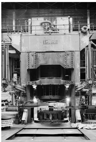
Hall 6 : vue générale de la presse Loire, 2 600 tonnes, emboutissant à froid. Phot. Thierry Petitberghien IVR31_20025901418X
