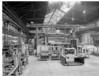
Hall 7 : le four de la presse de 1 500 tonnes. Vue de face. Phot. Thierry Petitberghien IVR31_20025901399V
