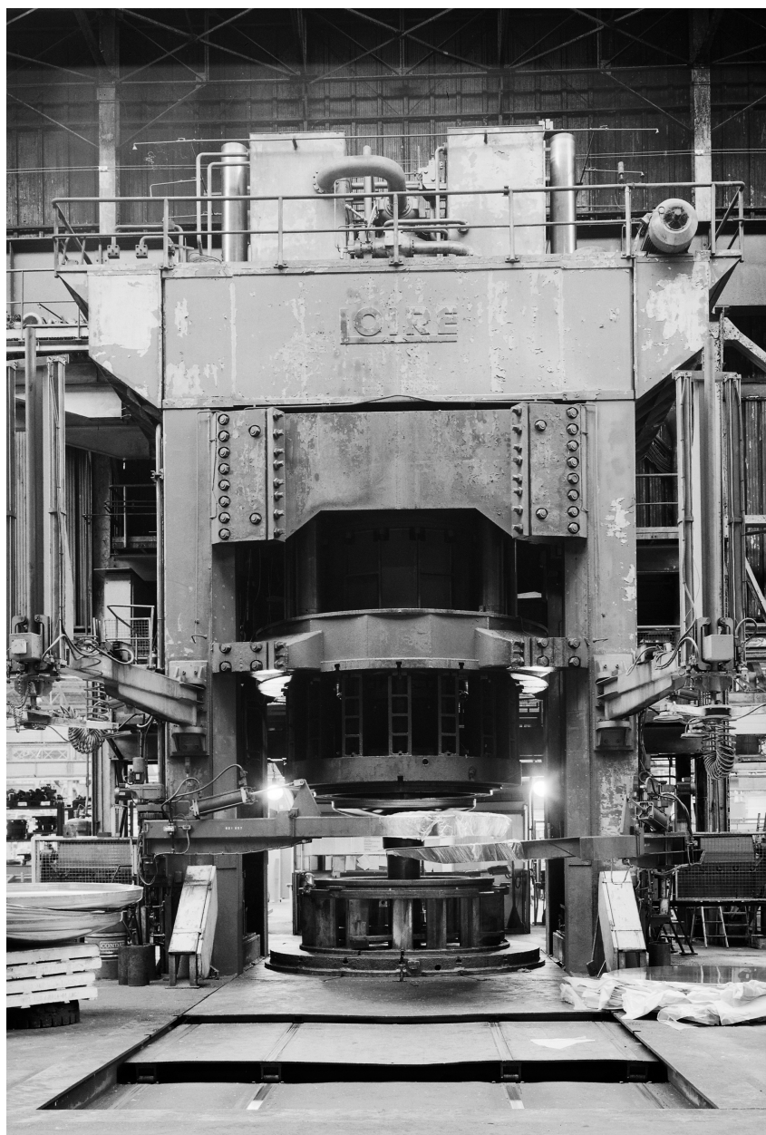
Hall 6 : vue générale de la presse Loire, 2 600 tonnes, emboutissant à froid.
