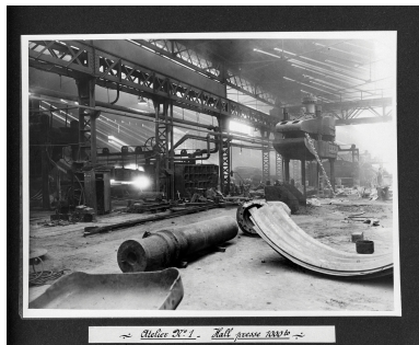
Atelier n° 1 : le hall de presses 1 000 tonnes, 16 février 1940. Photographe inconnu (coll. part., archives Cerec). Repro. Thierry Petitberghien IVR31_20025900597XB
