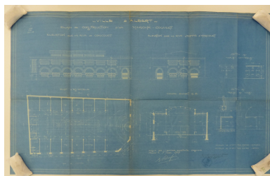
Ville d'Albert. Plan de construction d'un marché couvert. André Dufau architecte, 1927 (AD Somme ; 99O 153). Phot. Isabelle Barbedor IVR32_20218005008NUCA
