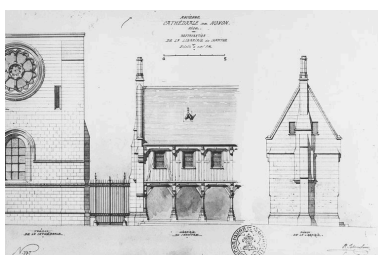
Projet de restauration. Elévation, par Seltersheim, 1875. Repro. Monnehay-Vulliet Marie-Laure IVR22_20096000464NUCA
