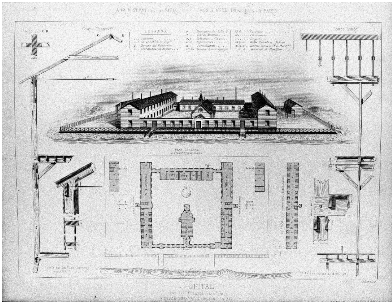
Vue cavalière générale en regardant depuis l'ouest, plan de distribution générale du rez-de-chaussée, plan de distribution du 1er étage de l'aile droite, coupes partielles des structures porteuses avec le détail des assemblages. Extrait de HUSSON, Armand. Étude sur les hôpitaux considérés sous le rapport de leur construction, p 130-131.
