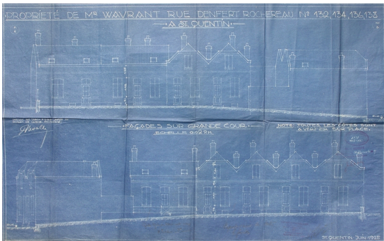
Elévations et coupes des logements sur cour, par R. Chevallier, 1925 (AC Saint-Quentin).
