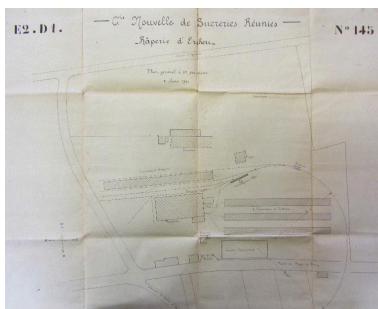
Plan masse de situation des bâtiments de la râperie, 2 août 1921 (AD Somme ; 5 M 524). Phot. Fournier Bertrand (reproduction) IVR22_20158006375NUCA
