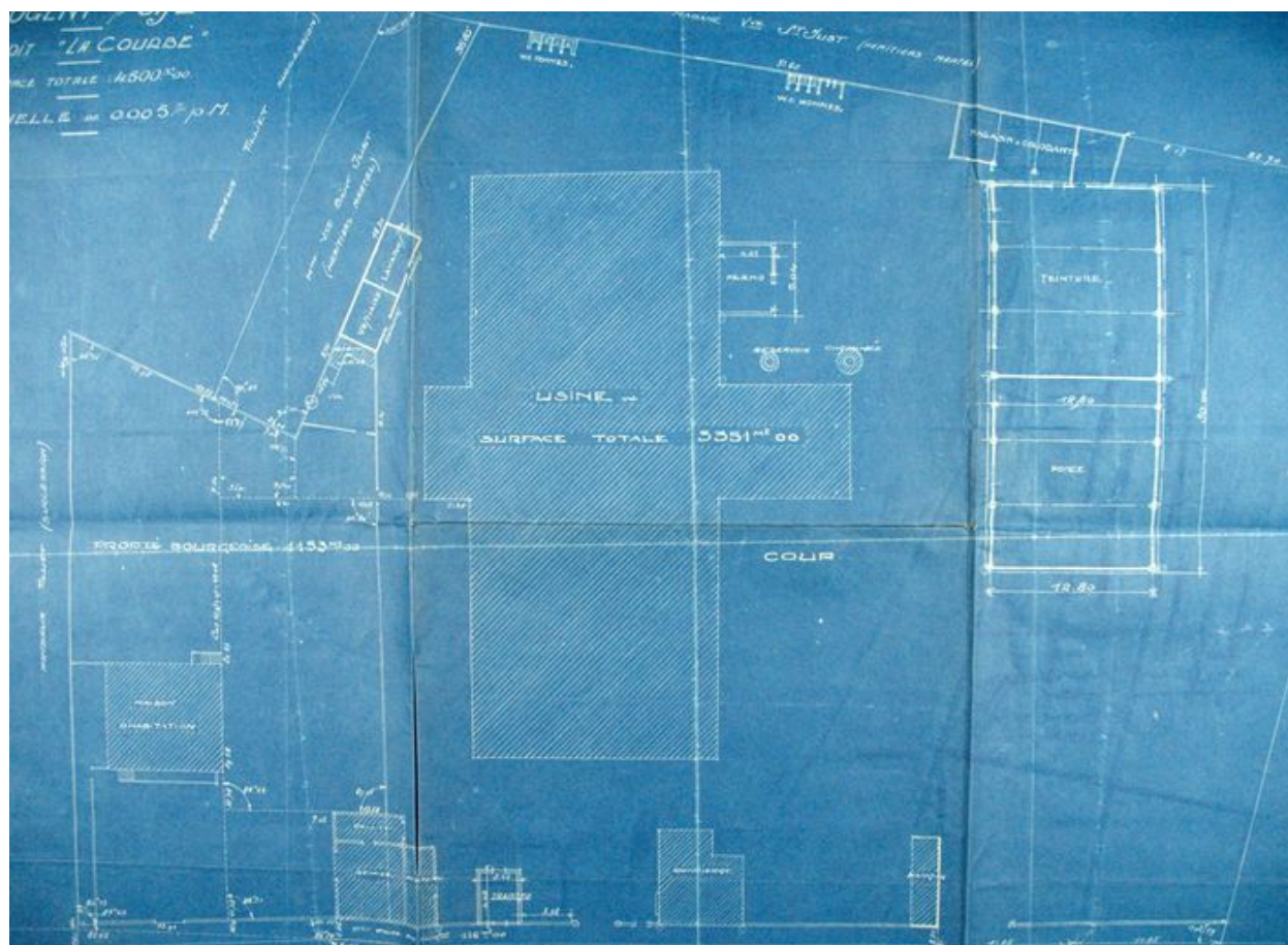
Plan de l'usine de fabrication de feutre, 1926 (AD Oise ; 5Mp2519).
