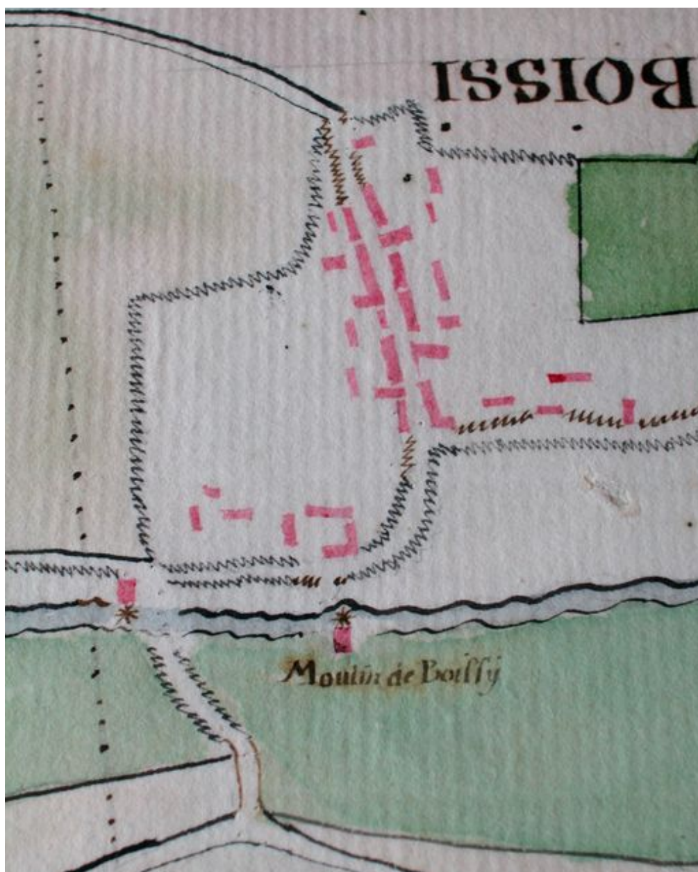
Plan du moulin à tan de Boissy, extrait du plan d'intendance de Roy-Boissy, Devert (arpenteur), 1785.
