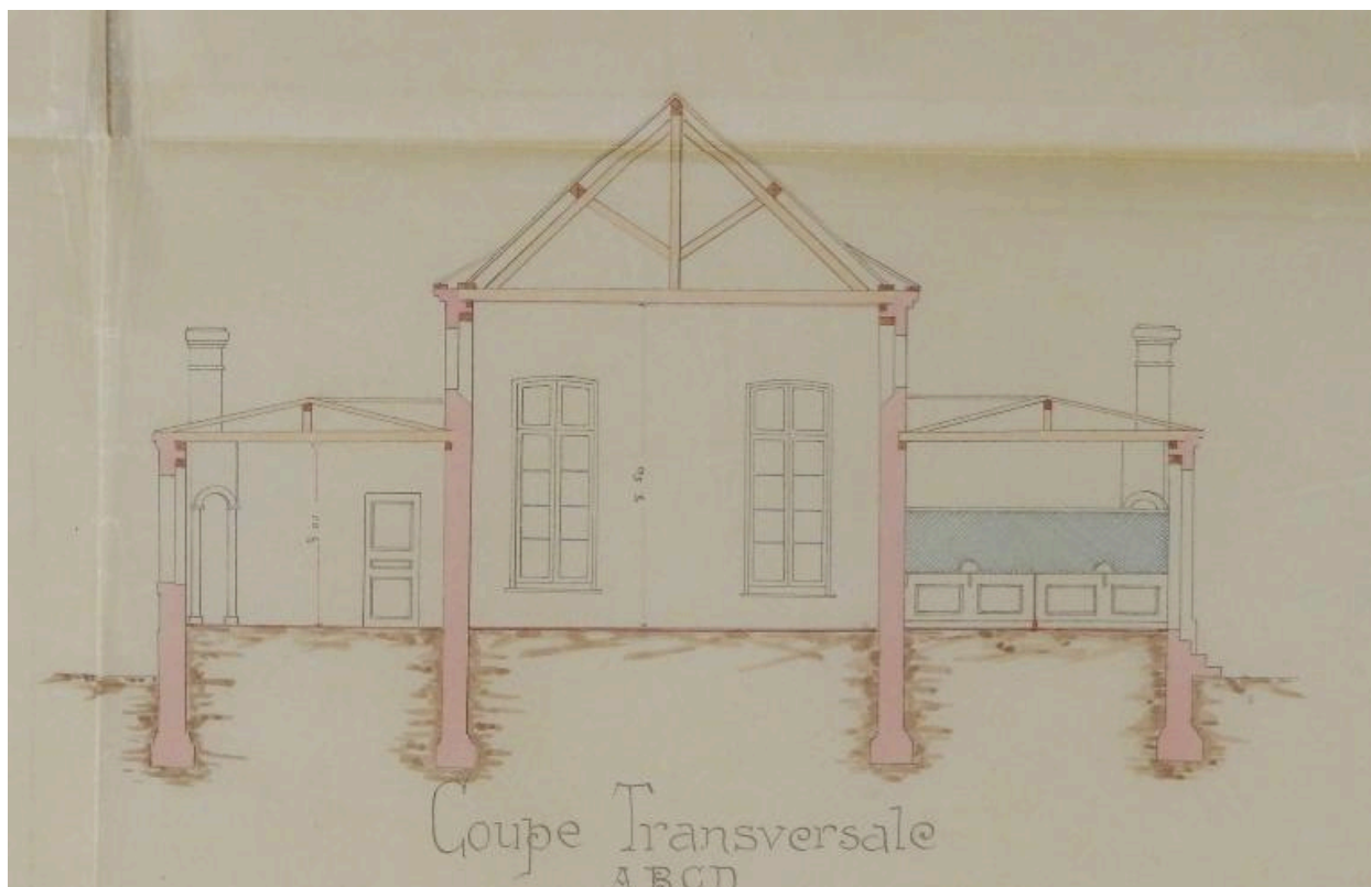
Coupe transversale, dressé par l'architecte Dingeon, 1880.
