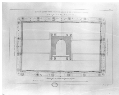
Plan, dessin par Nicolas Carnevali, gravé par Gaetano Cottafavi, in Barbier de Montault (X.). Description du maître-autel..., Rome, 1864, pl. I. Repro. Philippe Dapvri IVR31_19886200498X
