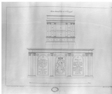
Elévation latérale 1, dessin par Nicolas Carnevali, gravé par Gaetano Cottafavi, in Barbier de Montault (X.). Description du maître-autel..., Rome, 1864, pl. IV. Repro. Philippe Dapvri IVR31_19886200496X
