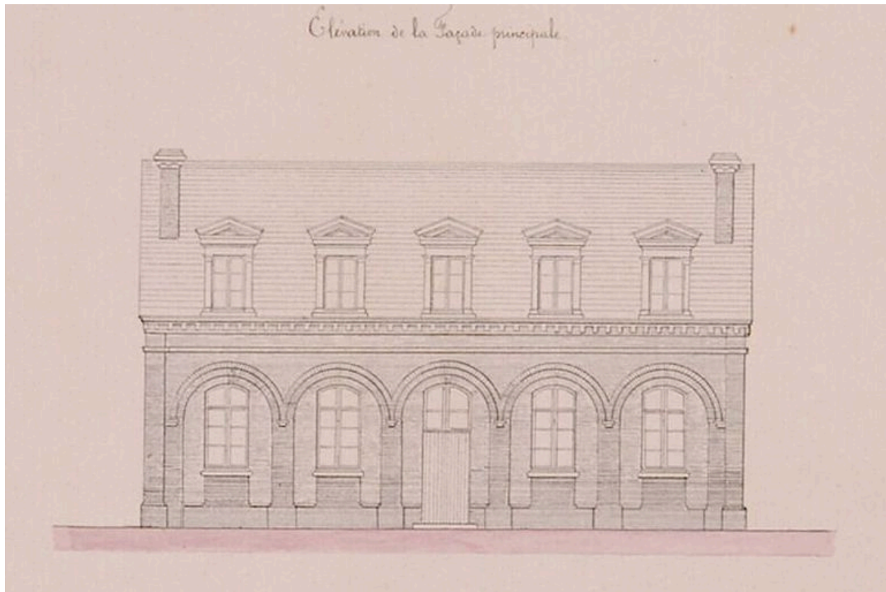
Élévation de la mairie-école, 1878 (AD Somme ; 99 T 3805 374).
