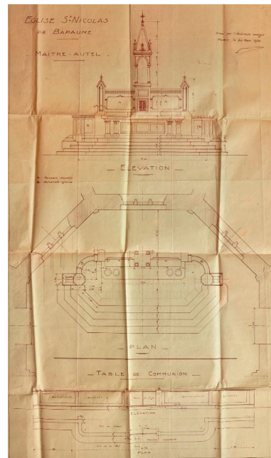
Église Saint-Nicolas de Bapaume - Maître-autel : élévation, plan. Daté et signé, Eugène Bidard, 20 mars 1933. (AD Pas-de-Calais, 10R21/52). Phot. Thibaut Pierre (reproduction) IVR32_20216200072NUCA
