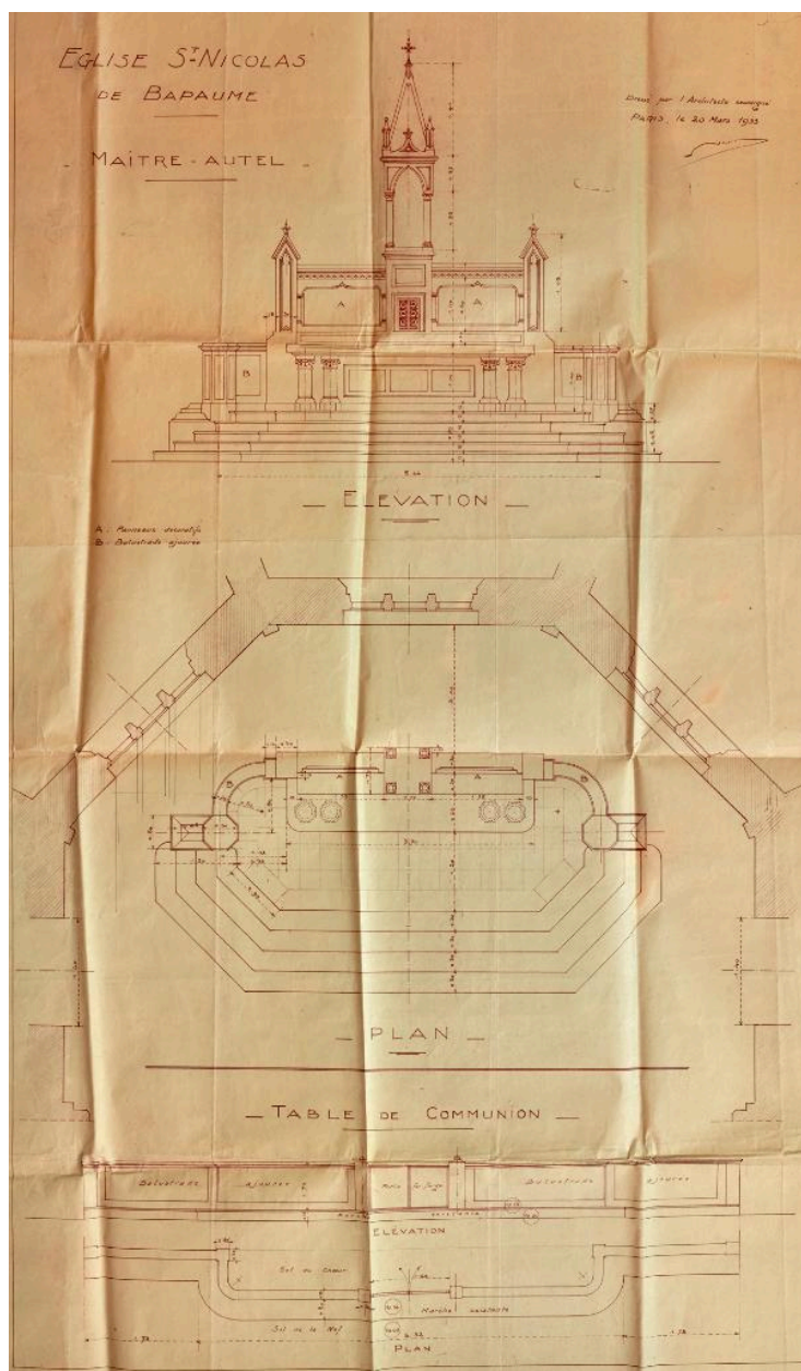
Église Saint-Nicolas de Bapaume - Maître-autel : élévation, plan. Daté et signé, Eugène Bidard, 20 mars 1933. (AD Pas-de-Calais, 10R21/52).
