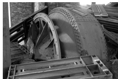
Broyeur à galets. Phot. Benoît Dufournier IVR22_19888000287Z
