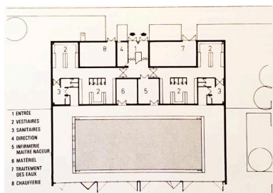
Plan schématique de la piscine Plein Soleil (publié dans la revue Piscines, n°31, 1971). Phot. Laurence Schlosser (reproduction) IVR32_20178005326NUCA
