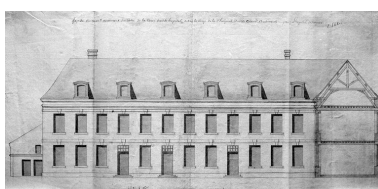
Projet d'élévation, par Mouton, 1775 (BM Noyon ; E 56 bis). Phot. Martine Plouvier (reproduction) IVR22_19876000369Z
