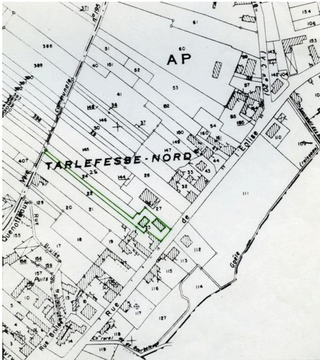
Plan de situation. Extrait du plan cadastral de 1974, section AP 23.
