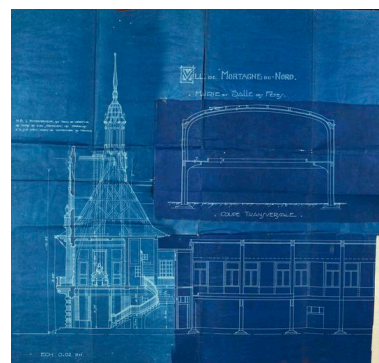
Coupe et jonction avec la salle des fêtes, Fernand Baud et Marcel Coquet architectes, 1925 (AD Nord 20421/197). Phot. Hubert Bouvet IVR31_20105900578NUCA
