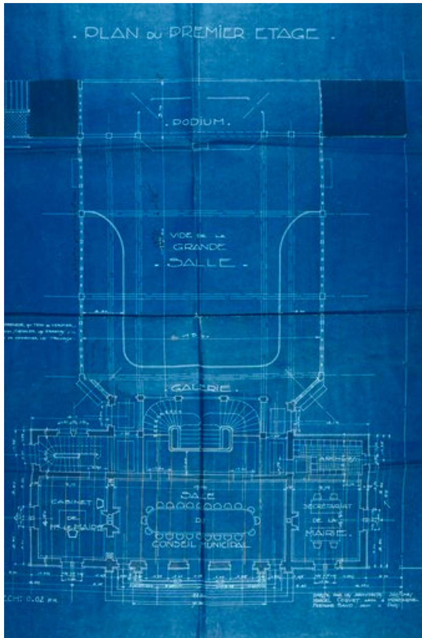
Plan du premier étage, Fernand Baud et Marcel Coquet architectes, 1925 (AD Nord 20421/197).
