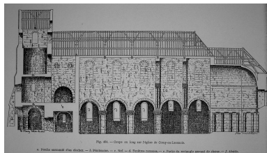
Coupe de l'église en 1879 (FLEURY, Edouard, p.26). Repro. Inès Guérin IVR22_20030203047NUCAB
