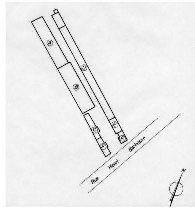
Schéma de situation : A. Fonderie, B. Atelier de fabrication, C. Cantines, écuries, D. Ateliers et magasins, E. Bureau, F. Logements. Dess. Monnehay-Vulliet Marie- Laure , Autr. Stéphane Gonet IVR22_20158001090NUD
