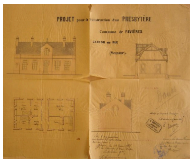
Plan, coupe et élévation du projet de construction du presbytère en 1865.
