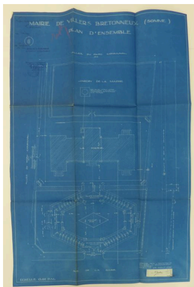
Projet de reconstruction de l'église de Villers-Bretonneux. Somme. Plan d'ensemble. Tirage de plan, A. Guilbert architecte, 23 août 1926 (AD Somme ; 990 3737). Phot. Isabelle Barbedor IVR32_20208005193NUCA
