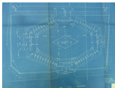
Projet de reconstruction de l'église de Villers-Bretonneux. Somme. [Plan du square]. Tirage de plan, A. Guilbert architecte, 23 août 1926 (AD Somme ; 990 3737). Phot. Isabelle Barbedor IVR32_20208005192NUCA
