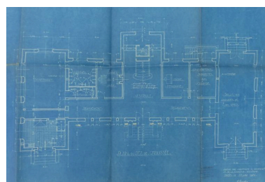
Projet de reconstruction de l'église de Villers-Bretonneux. Somme. Plan du rez-de-chaussée. Tirage de plan, A. Guilbert architecte, 22 juillet 1926 (AD Somme ; 990 3737). Phot. Isabelle Barbedor IVR32_20208005190NUCA
