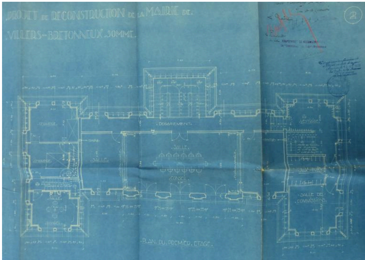
Projet de reconstruction de l'église de Villers-Bretonneux. Somme. Plan de l'étage. Tirage de plan, A. Guilbert architecte, 22 juillet 1926 (AD Somme ; 990 3737).
