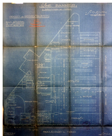
Usine Pannier. Projet de reconstruction B, par Dumortier, 1920 (AC Saint-Quentin). Phot. Pillet Frédéric IVR22_20040200651NUCAB
