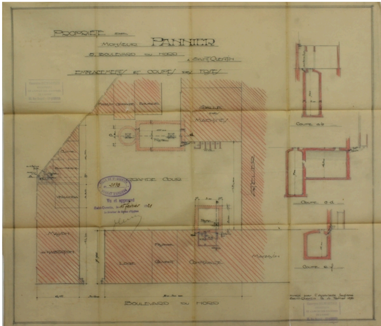
Usine Pannier. Plan partiel, par Dumortier, 1921 (AC Saint-Quentin).
