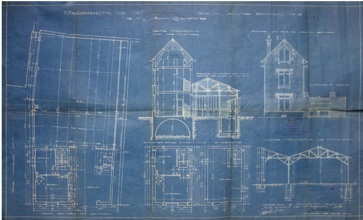
Projet d'atelier des architectes Hue et Thill, 1922 (abandonné). (AC Saint-Quentin).
