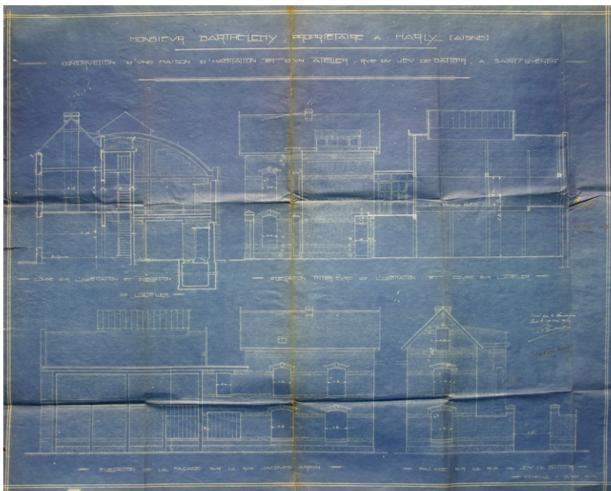
Façades et coupes, par Roulaux, 1922 (AC Saint-Quentin).
