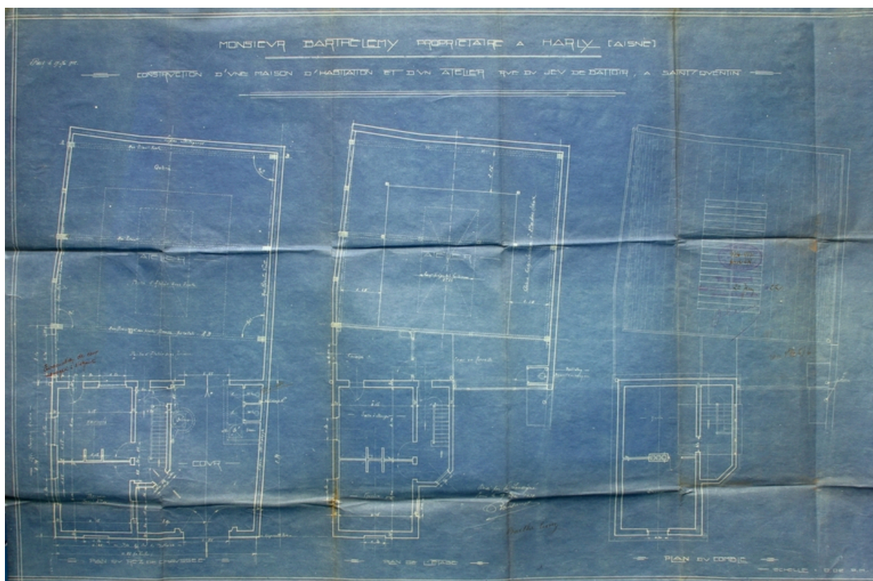
Plans par niveau, par Rouleaux, 1922 (AC Saint-Quentin).
