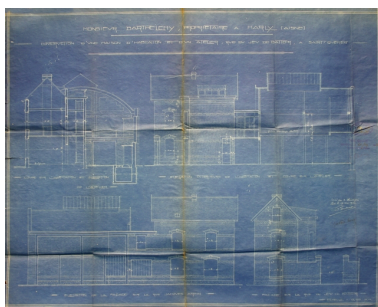
Façades et coupes, par Rouleaux, 1922 (AC Saint-Quentin). Phot. Pillet Frédéric IVR22_20050206448NUCAB
