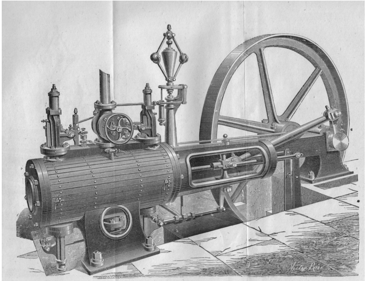
Machine à vapeur Zimmermann construite par Lecoite & Villette, présentée à l'Exposition Universelle de 1878 (Bulletin de la Société Industrielle de Saint-Quentin et de l'Aisne).
