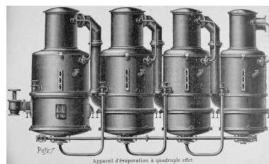
Appareil d'évaporation à quadruple effet, vers 1900 (Le département de l'Aisne à l'Exposition Universelle de Paris en 1900). Phot. Pillet Frédéric IVR22_20050206025NUCAB
