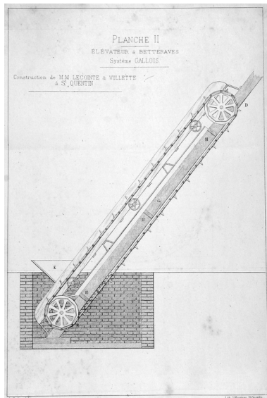
Elévateur à betteraves Système Gallois construit par Lecoite et Vilette, 1878-1880 (Bulletin de la Société Industrielle de Saint-Quentin et de l'Aisne). Phot. Pillet Frédéric IVR22_20050206022NUCAB
