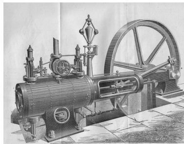
Machine à vapeur Zimmermann construite par Lecoite & Vilette, présentée à l'Exposition Universelle de 1878 (Bulletin de la Société Industrielle de Saint-Quentin et de l'Aisne). Phot. Pillet Frédéric IVR22_20050206029NUCAB
