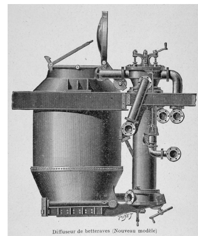
Diffuseur de betteraves, vers 1900 (Le département de l'Aisne à l'Exposition Universelle de Paris en 1900). Phot. Pillet Frédéric IVR22_20050206026NUCAB
