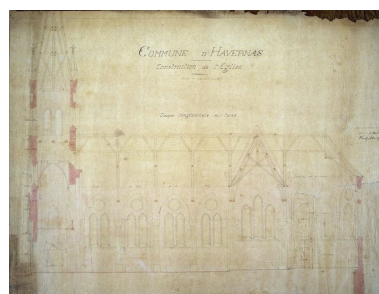
Coupe longitudinale ouest-est par Victor et Paul Delefortrie, 9 août 1872 (arch. privées). Phot. Monnehay-Vulliet Marie-Laure IVR22_20108000183XA
