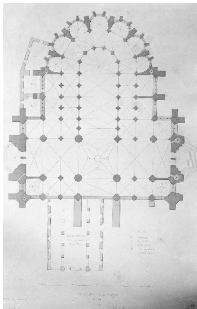
Plan de la cathédrale, 19e siècle. Phot. Laurent Jumel (reproduction) IVR22_19956000319XB
