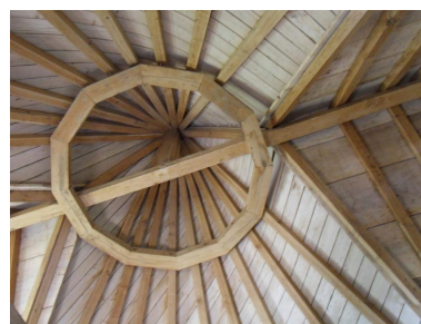
Vue de la charpente. Phot. Isabelle Barbedor IVR22_20108010158NUCA
