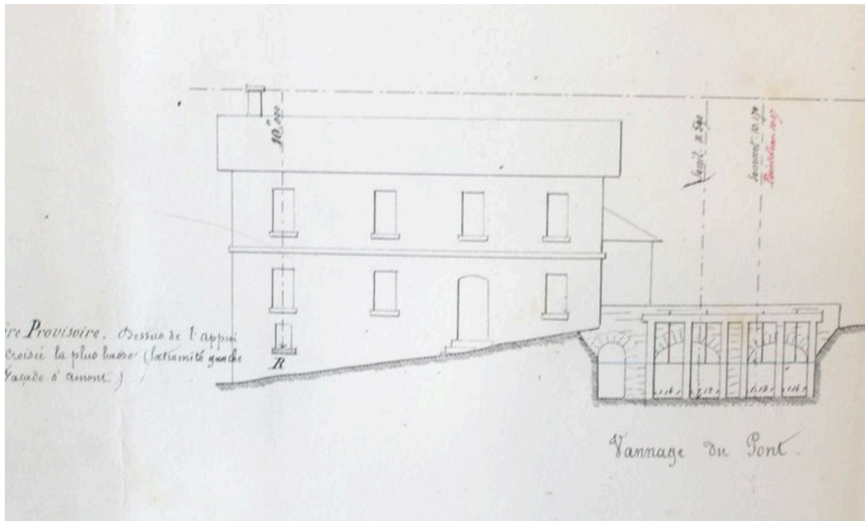
Elévation du moulin, 2 juillet 1856 (AD Oise ; 7Sp 142).
