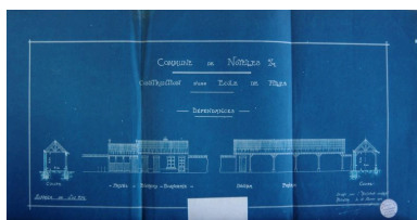
Coupe et élévations des dépendances du projet de la nouvelle école de filles par Alfred Marchand, en 1913. Phot. Inès Guérin IVR22_20068005046NUCAB
