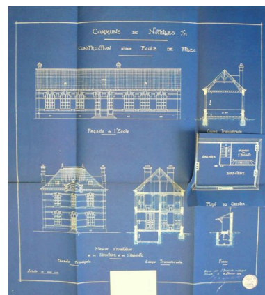
Projet de construction de la nouvelle école et de l'habitation de l'institutrice par Alfred Marchand, en 1913, plan, coupe et élévation. Phot. Inès Guérin IVR22_20068005044NUCAB
