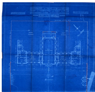
Plan d'ensemble de l'école de filles en 1929. Phot. Monnehay-Vulliet Marie-Laure IVR22_20068000006XAB
