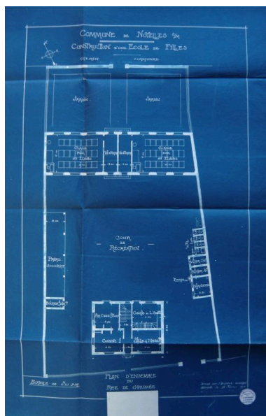
Plan d'ensemble du projet de construction d'une nouvelle école de filles, par Alfred Marchand, en 1913. Phot. Inès Guérin IVR22_20068005045NUCAB
