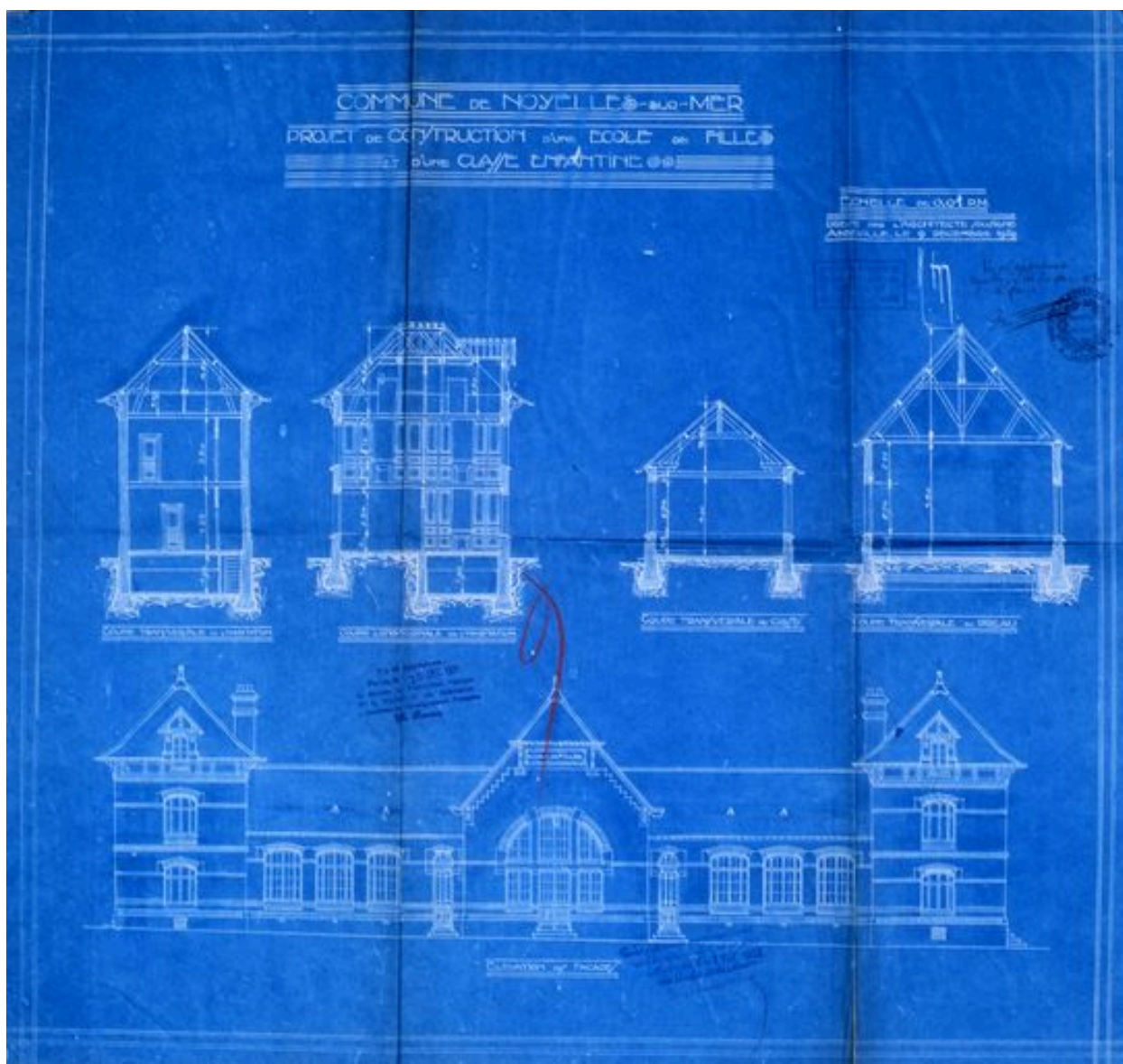
Coupe et élévation de l'école de filles.
