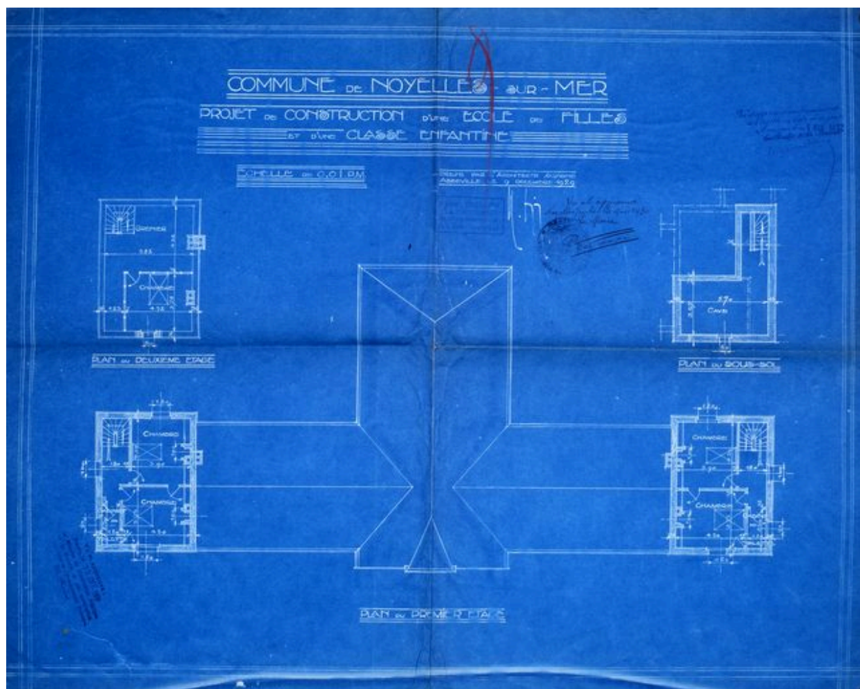
Plan du premier étage de l'école des filles.
